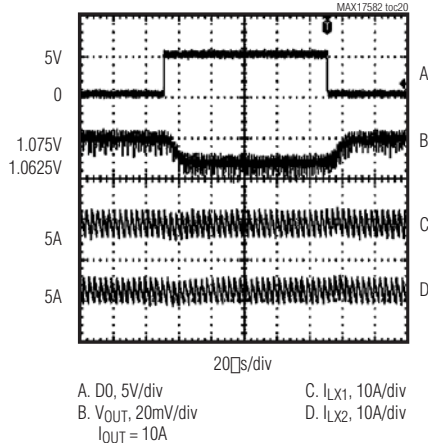
DYNAMIC VID CODE CHANGE (DO = 12.5mV)
