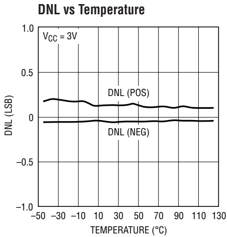
2656 G04
