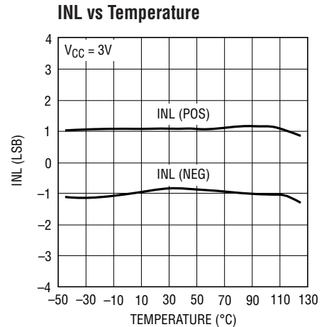
2656 G03
