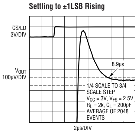
2656 G06
