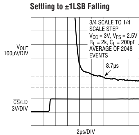
2656 G07
