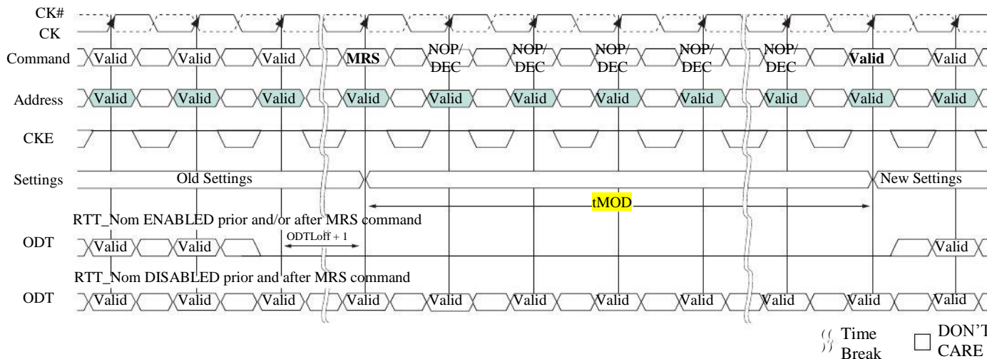
Figure 2.3.1b tMOD Timing
