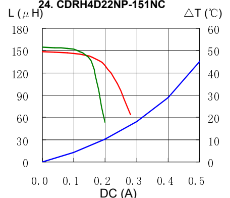
24. CDRH4D22NP-151NC
