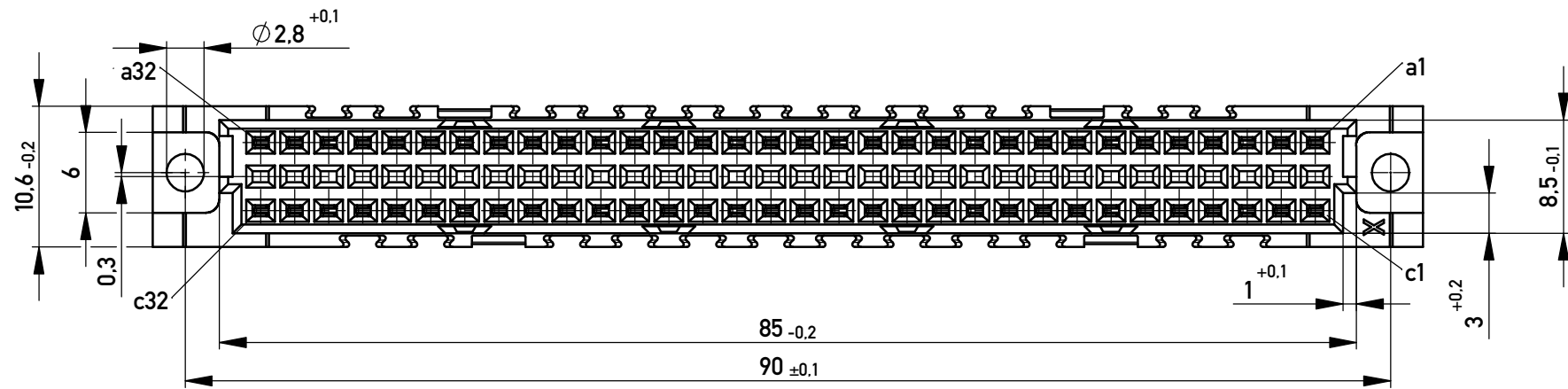
Bestückungsplan / contact layout
