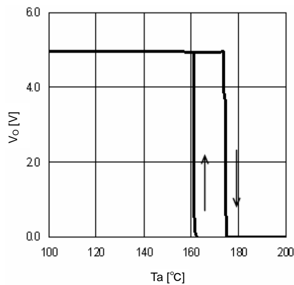
Fig.28 TSD ( I_o=0\text{mA} )
