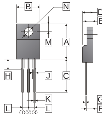
ITO-220
