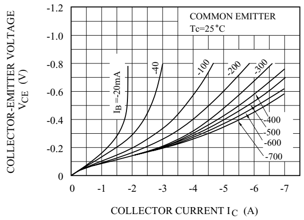
V_{CE} - I_C
