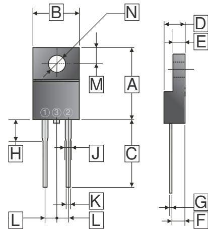
ITO-220A
