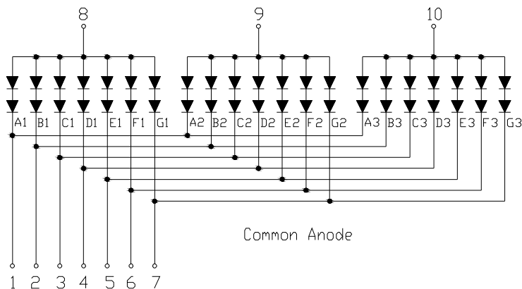
FYA-CR41BX
