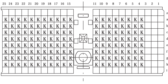
Lochbild für Leiterplatte (Bestückungsseite)
