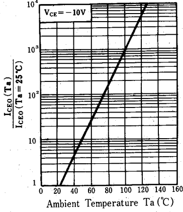
I_{CE0} - T_a
