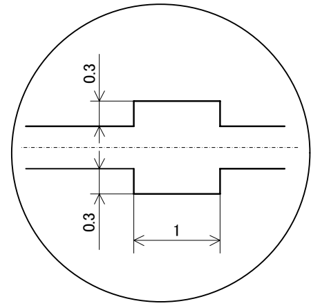
ストップパー部詳細図 Detail of stopper
