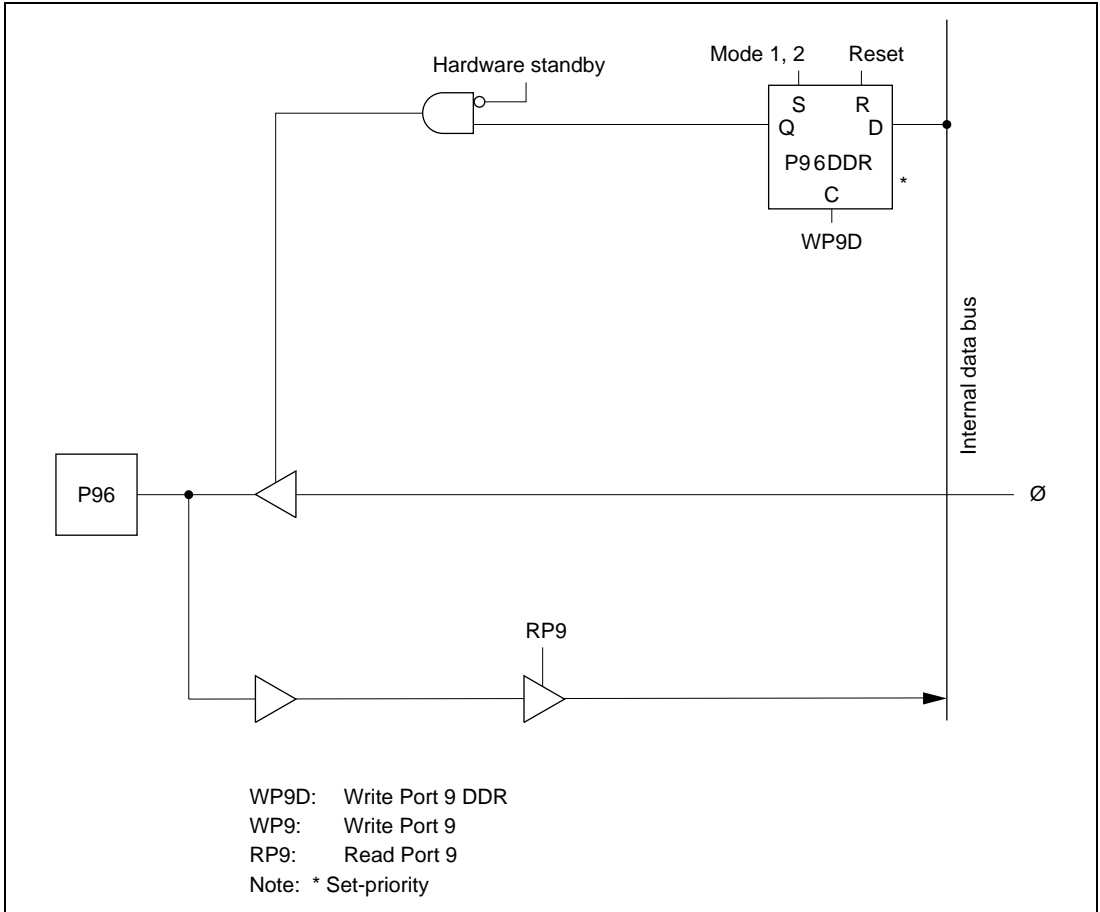
Figure 6.9 (d) Port 9 Schematic Diagram (Pin P9 6 )
