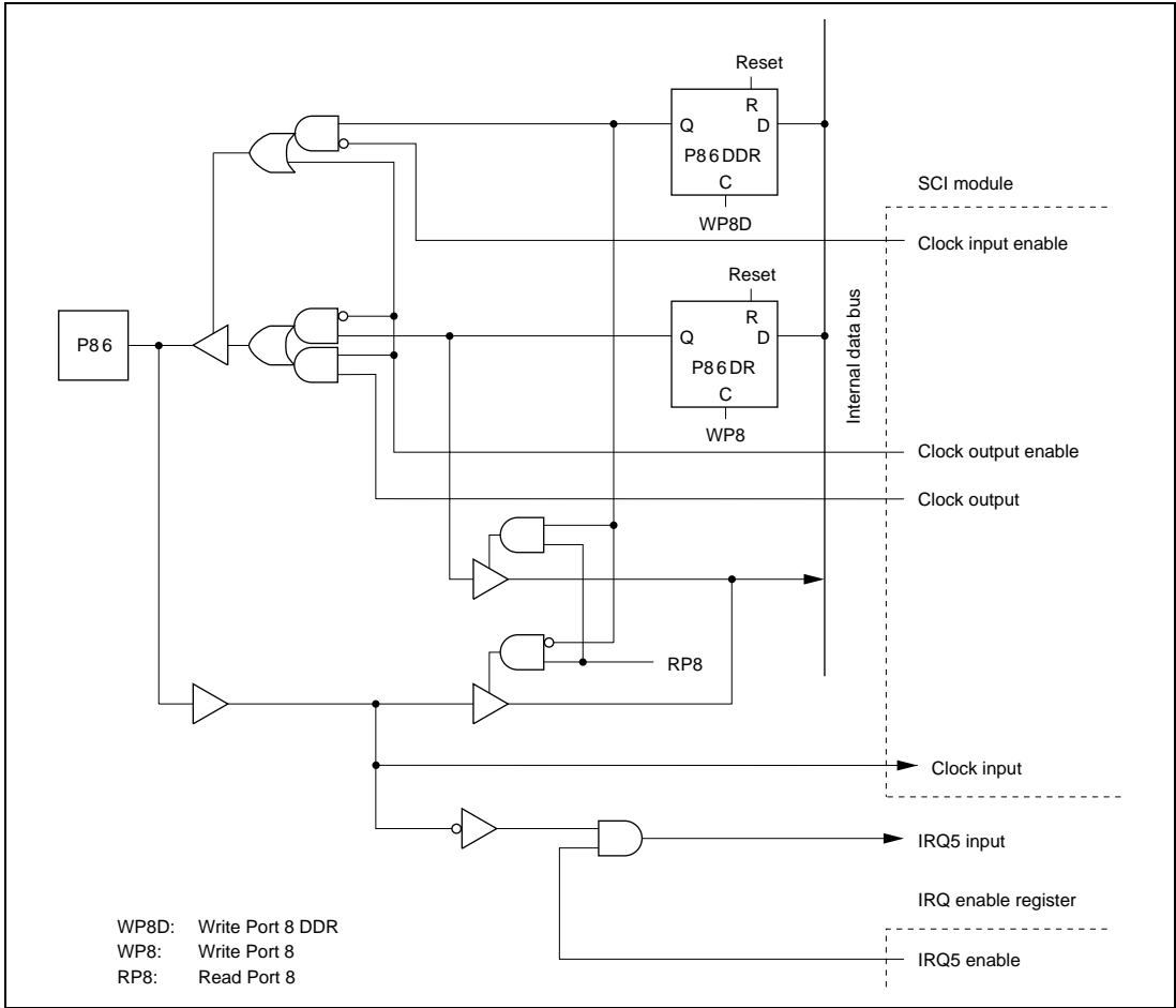
Figure 6.8 (d) Port 8 Schematic Diagram (Pin P8 6 )
