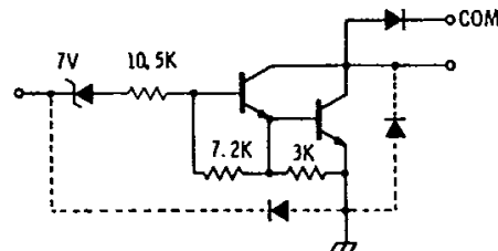
Dwg. No A-9650
