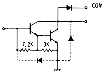
Dwg. No A-9595
