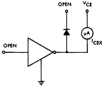
Dwg. No. A-9729A
