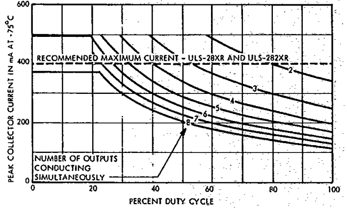
Dwg. No. A-10,871A
