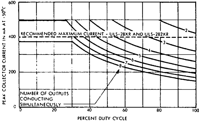
Dwg. No. A-10,870A
