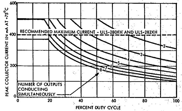
Dwg. No. A-10,876A
