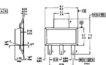
SOT-223
