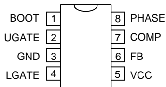
SOP-8 (APW7065C)
