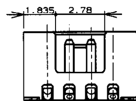
4極 4 Pos. (SCALE 5-1)
