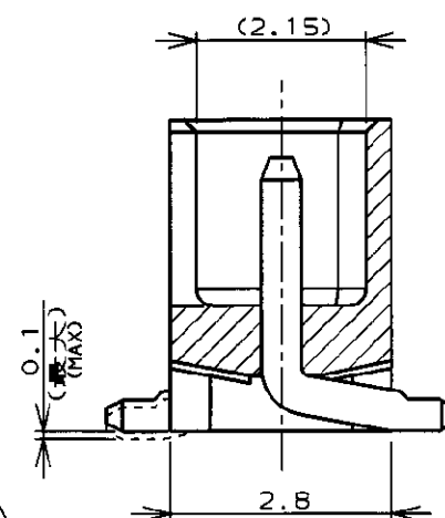
20極 20 Pos. (SCALE 5-1)
