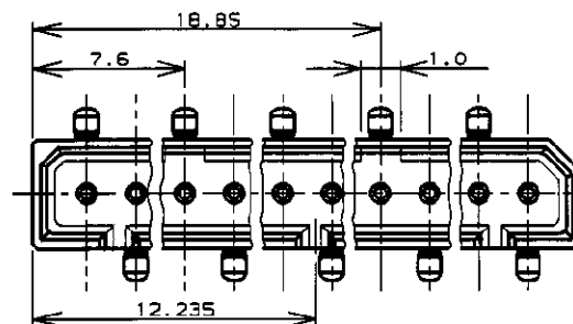
20極 20 Pos. (SCALE 5-1)
