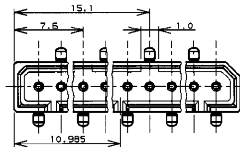
17極 17 Pos. (SCALE 5-1)
