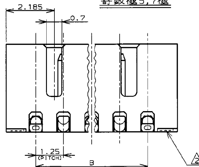
ODD NUMBER Pos. 5, 7 Pos. 奇数極 5, 7極
