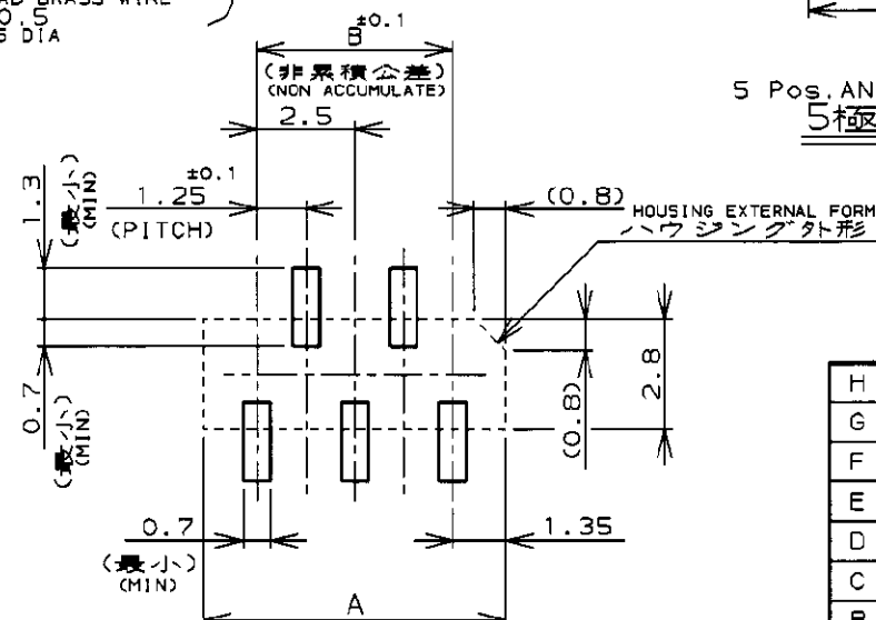
P.C.B MOUNTING LAYOUT 基板加工寸法 (適用基板厚: 0.6mm最小) (APPLICABLE P.C.B THK: 0.6mm MIN)
