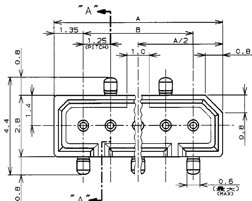
ODD NUMBER Pos. 5, 7 Pos. 奇数極 5, 7極
