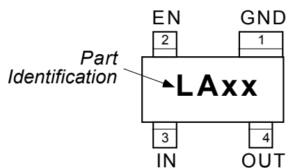
SOT-143 (M4)
