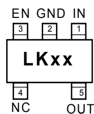
SOT-23-5 (M5)
