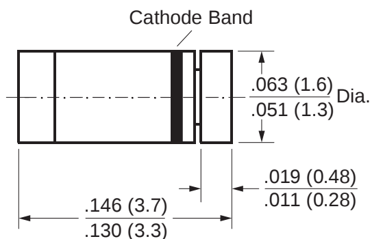
MiniMELF (SOD-80C)
