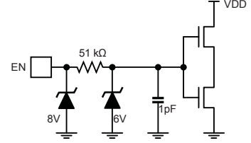
Figure 19d. EN Input
