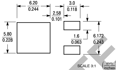
DPAK
