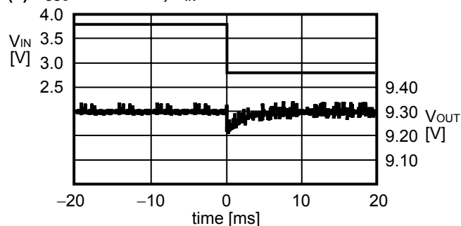
(4) f_{OSC} = 700\text{ kHz} , V_{IN} = 3.8\text{ V} \rightarrow 2.8\text{ V}
