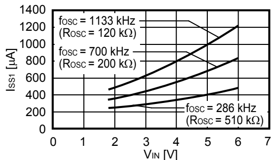
I_{SS} vs. V_{IN}
