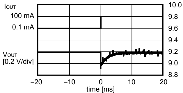
(5) f_{OSC} = 286\text{ kHz} , I_{OUT} = 0.1\text{ mA} \rightarrow 100\text{ mA}
