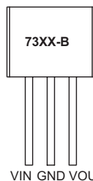
TO-92-B
