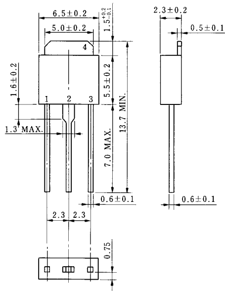
2SC3588
