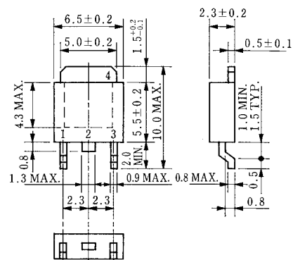
2SC3588-Z
