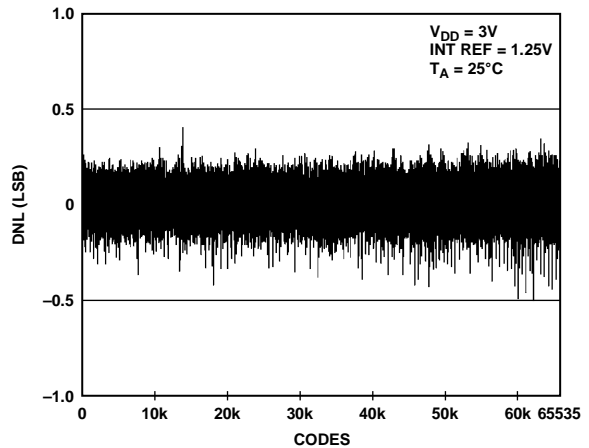
Figure 15. DNL AD5669R-1—Internal Reference
