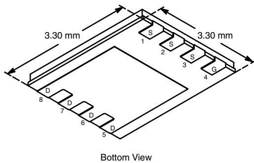
PowerPAK 1212-8
