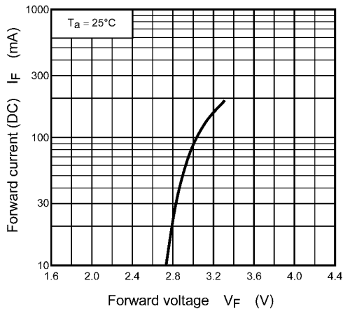
Fig. 8.1 I_F - V_F
