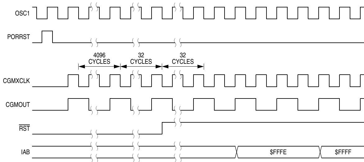
Figure 14-6. POR Recovery
