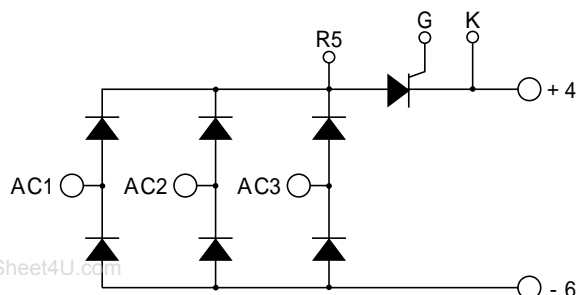
回路図 CIRCUIT
