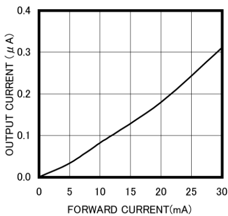
IF VS I o @VR=10V
