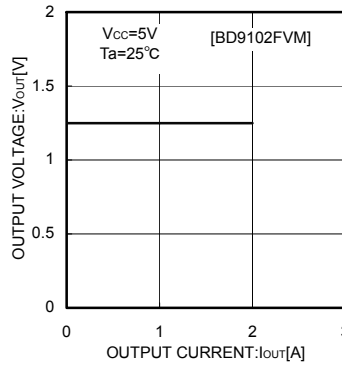
Fig.7 Iout-Vout
