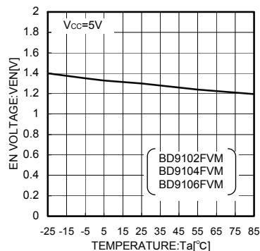
Fig.34 Ta-VEN
