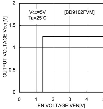
Fig.4 Ven-Vout
