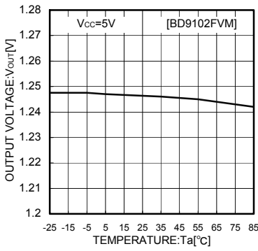
Fig.25 Ta-VOUT
