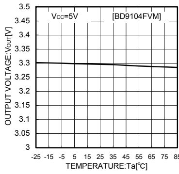
Fig.26 Ta-VOUT
