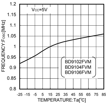
Fig.31 Ta-Fosc
