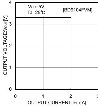
Fig.8 Iout-Vout
