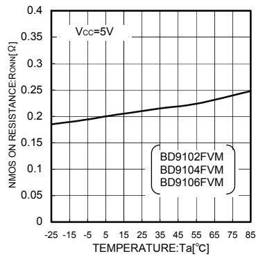
Fig.32 Ta-RONN
