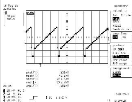
Ref.3 Y separated output : IC300, #96
