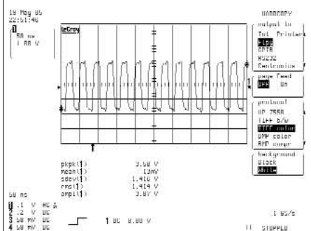
Ref.4 ITU 656 Clock out : IC200, #83
