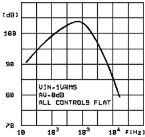
通道隔离 vs 频率
