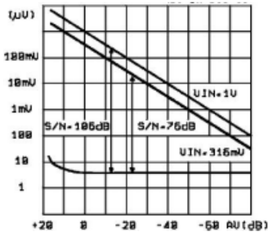
信噪比 vs 音量
