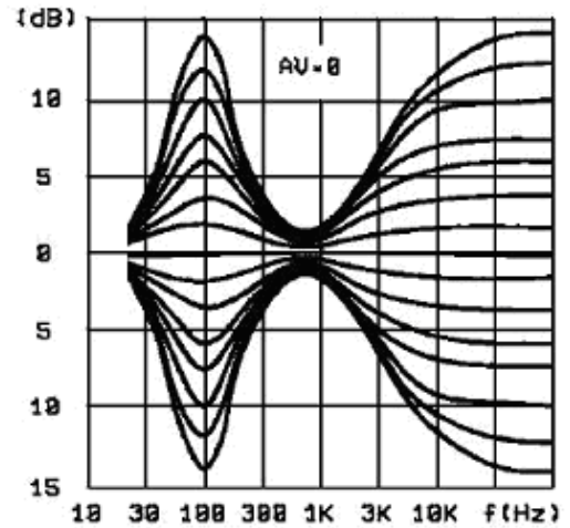
频率特性
