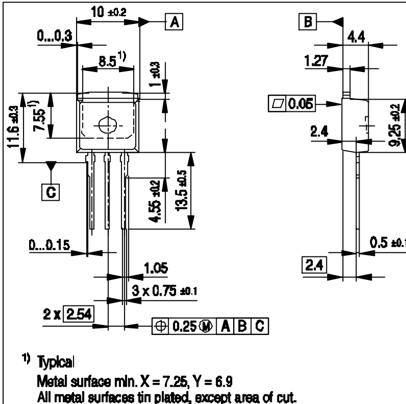
P-TO-262-3-1 (I 2 -PAK)
