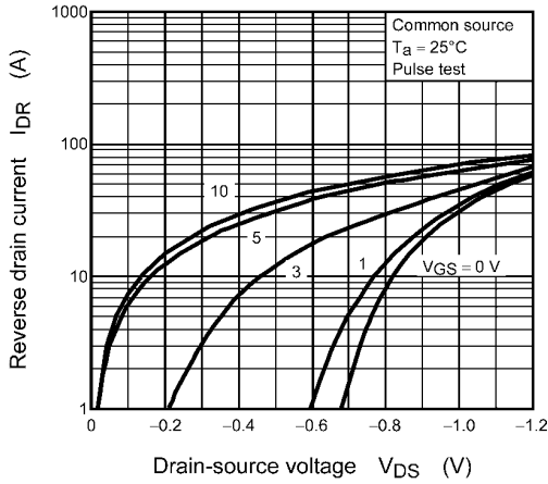
Fig. 9.7 I_{DR} - V_{DS}
