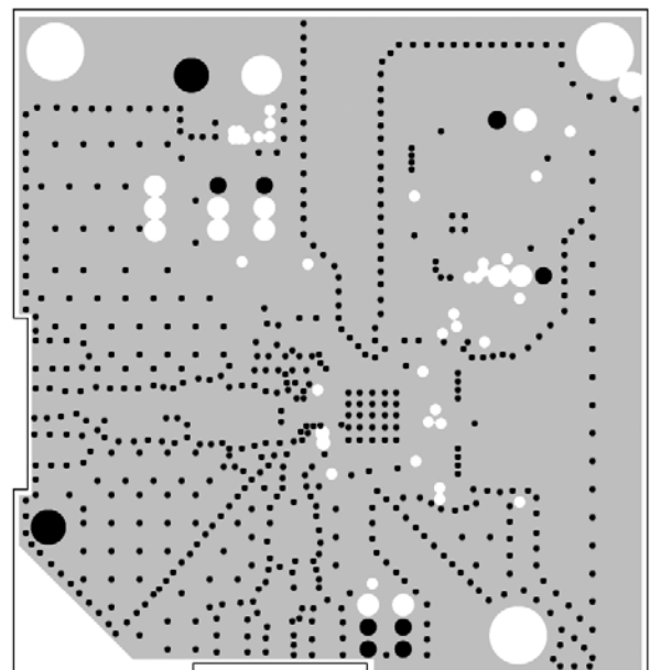
Inner Layer 3
