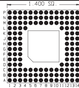
135 Pins Footprint 14011
