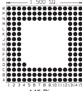
145 Pins Footprint 15024
