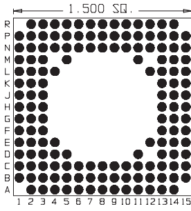
149 Pins Footprint 15019
