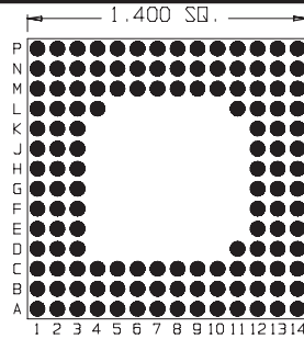
135 Pins Footprint 14012
