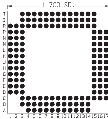
145 Pins Footprint 17004
