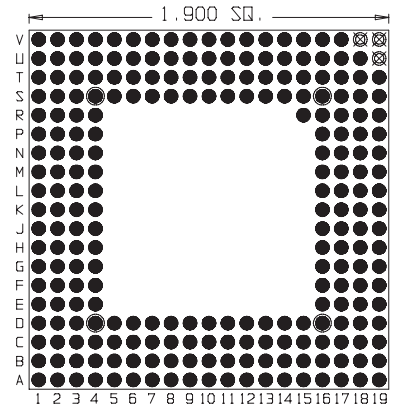
238 Pins Footprint 19007 - ZIF
