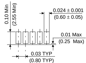
Detail Y
