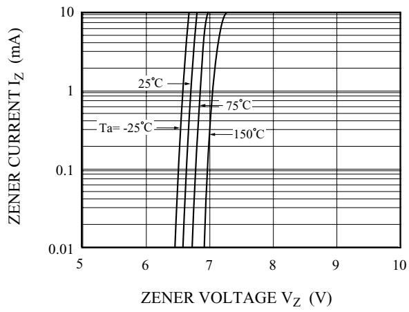
V_Z - I_Z
