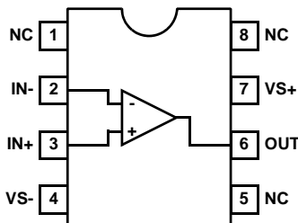
EL2126 (8 LD SO) TOP VIEW
