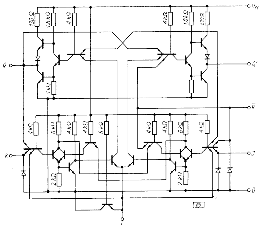
Schemat ideowy pojedynczego przerzutnika układu UCY74107N
