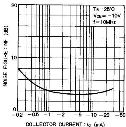
Fig. 12 雑音指数—コレクタ電流特性
