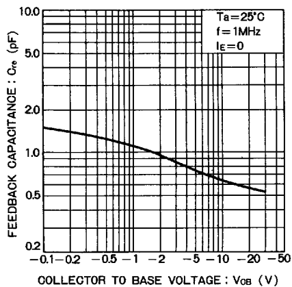
Fig. 8 帰還容量—電圧特性
