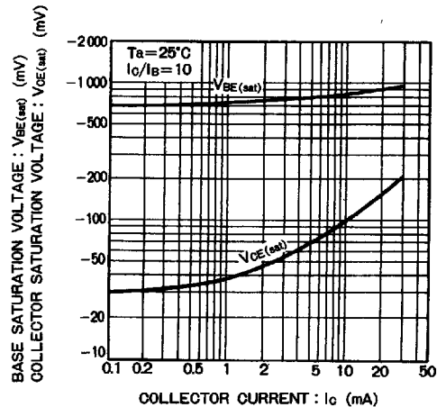
Fig. 6 ベース・エミッタ飽和電圧-コレクタ電流特性 コレクタ・エミッタ飽和電圧
