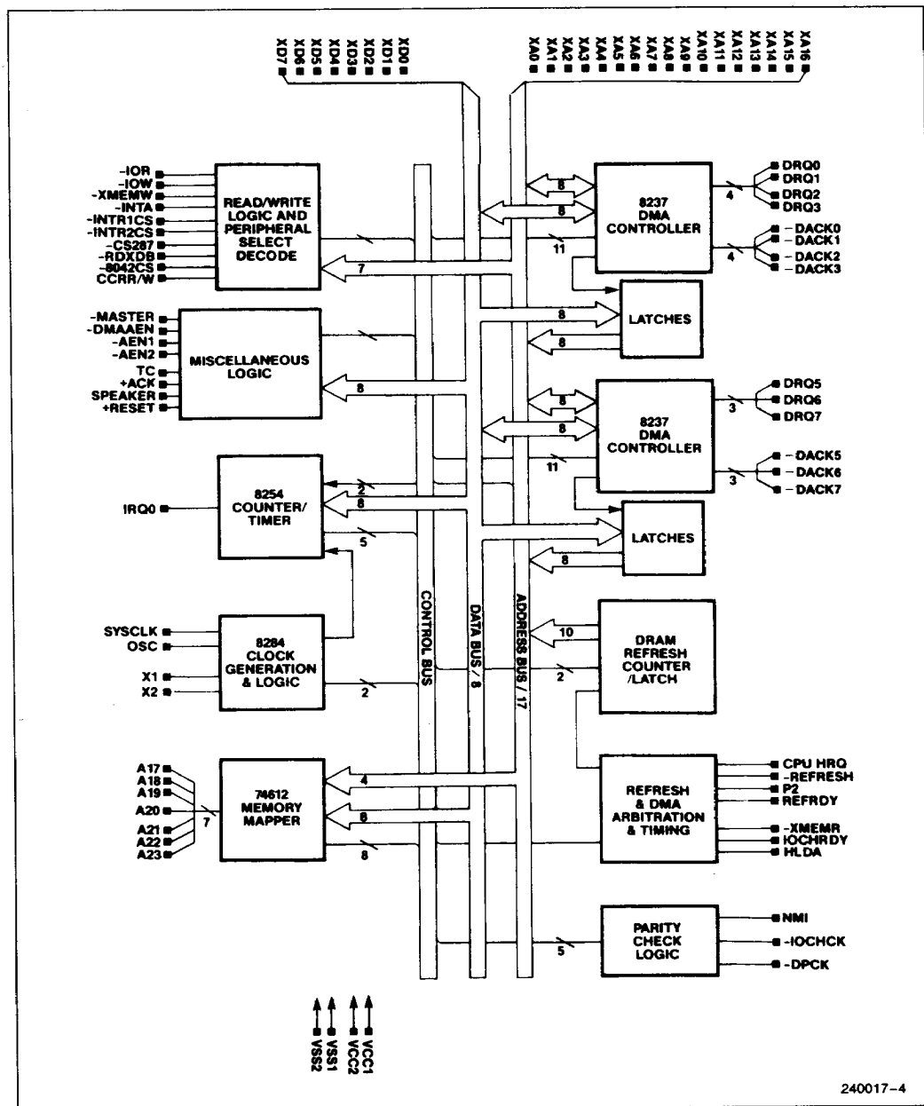
82231—Block Diagram
