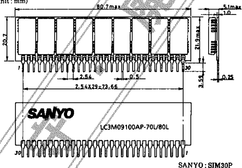
外形図 3186 リードタイプ (unit: mm)
