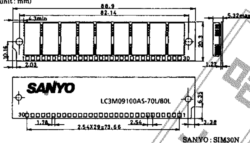
外形図 3185 ソケットタイプ (unit: mm)
