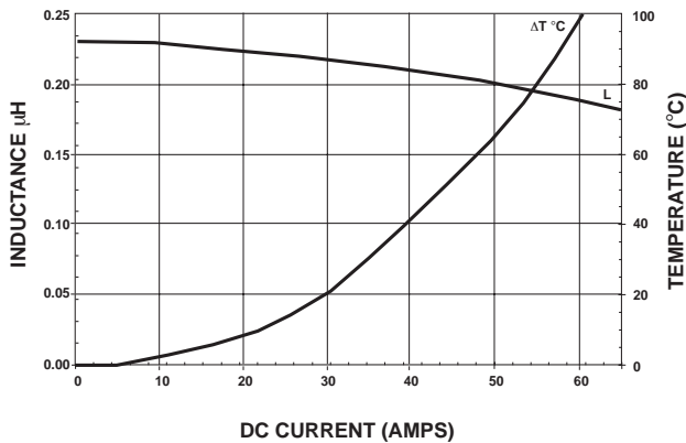
IHLP-5050CE-01 0.22 \mu H
