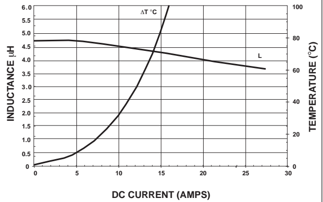
IHLP-5050CE-01 4.7 \mu H
