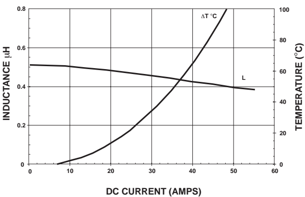
IHLP-5050CE-01 0.47 \mu H
