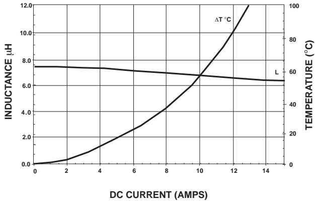
IHLP-5050CE-01 8.2 \mu H
