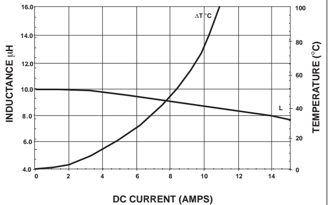
IHLP-5050CE-01 10 \mu H
