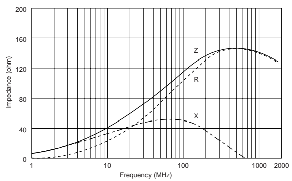
BLM18EG121SN1
