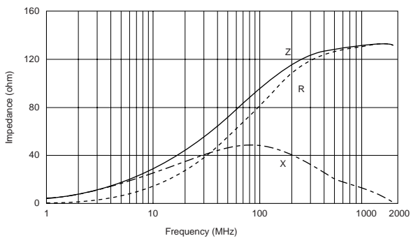
BLM18EG101TN1
