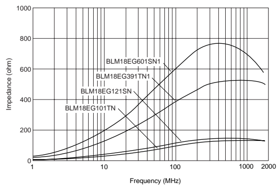
BLM18EG101TN1
