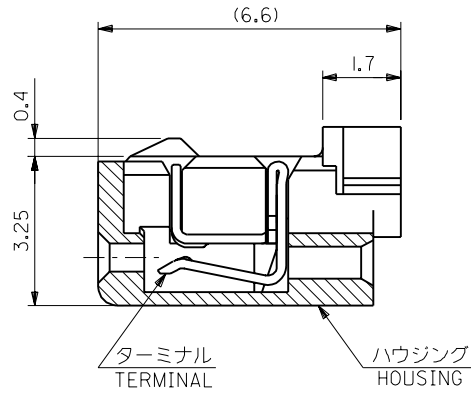
ターミナル装着状態図 FIGURE OF TERMINAL WHEN ASSEMBLED (SCALE : 10-1)
