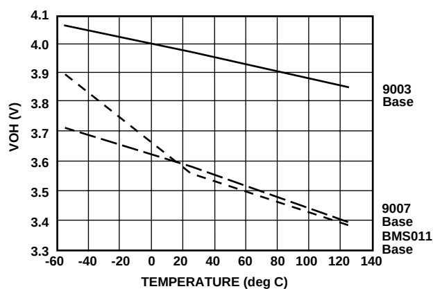
VOH Vs TEMP.
