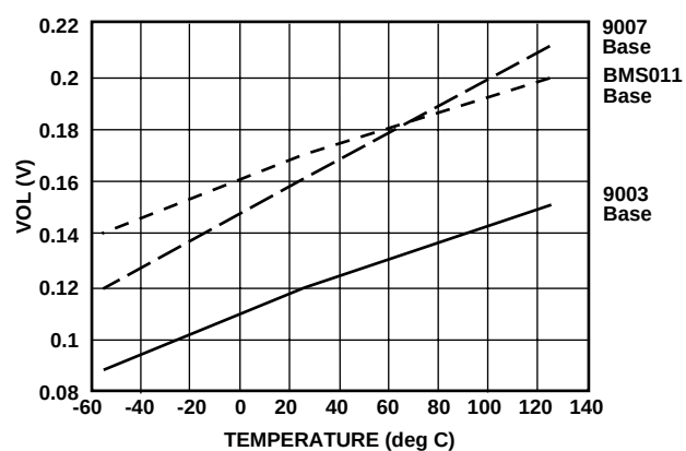
VOL Vs TEMP.
