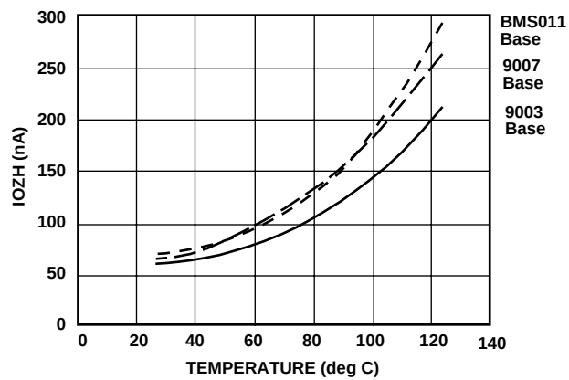
IOZH Vs TEMP.
