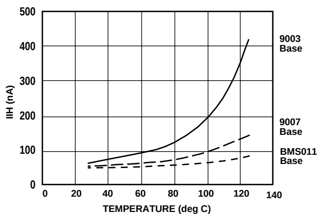
IIH Vs TEMP.
