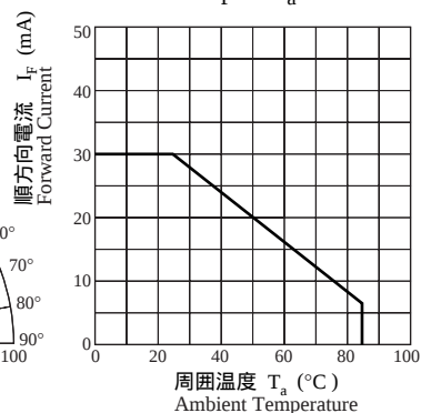
I_F - T_a
